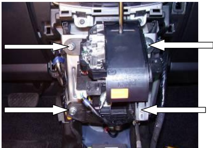
Открутить 4 штатных гайки селектора
