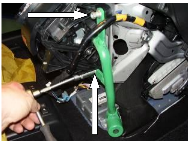
Закрутить 2 срывные гайки
