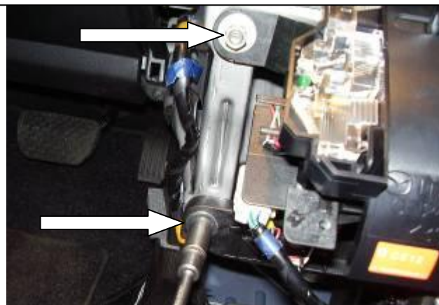
9 Заменить 2 штатные гайки на срывные 10
