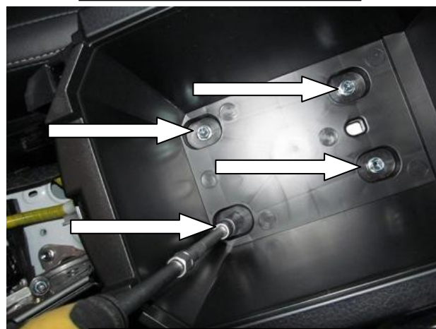
Открутить 4 самореза
