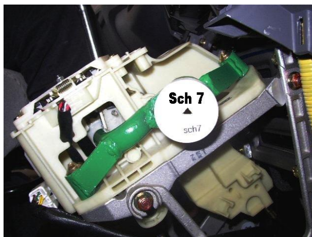
Разметить, используя разметочный шаблон, отверстие в консоли под корпус замка
