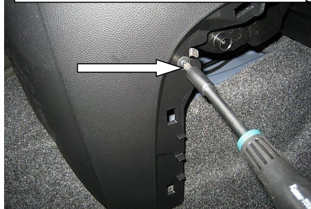
Открутить саморезы с обеих сторон
