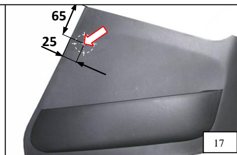
Разметить отверстие под корпус замка
