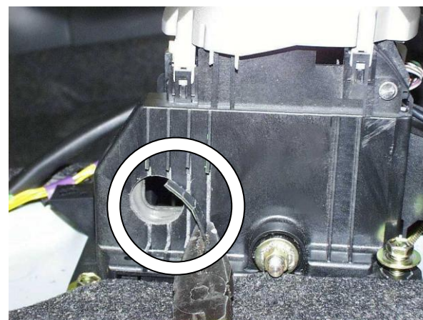
Удалить мешающие рёбра жёсткости
