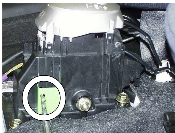
Просверлить отверстие в селекторе под ригель замка
