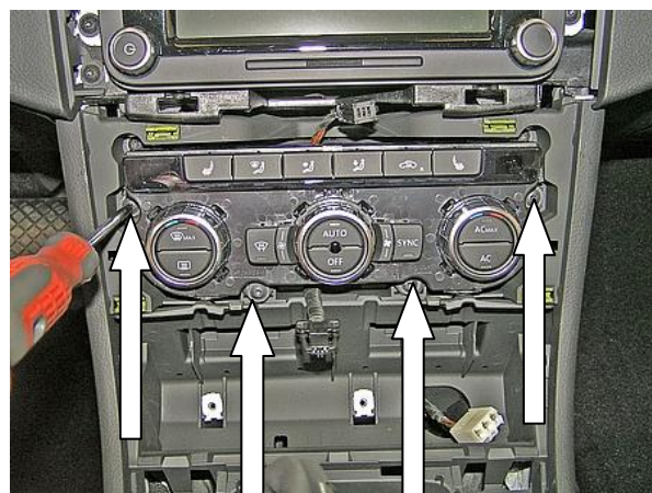
Открутить 5 саморезов
