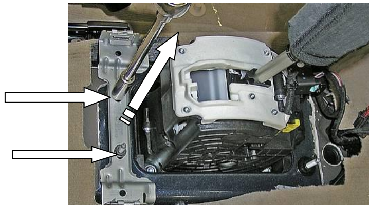
Открутить 2 штатные гайки селектора, снять держатель консоли
