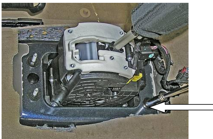
Открутить штатную гайку селектора
