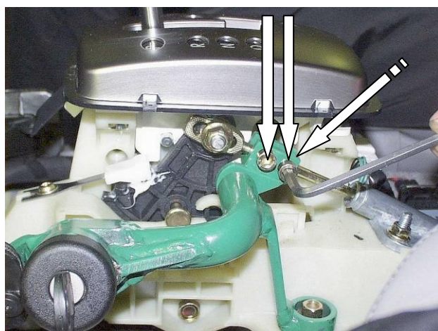
Установить хомут на тягу, зафиксировать
