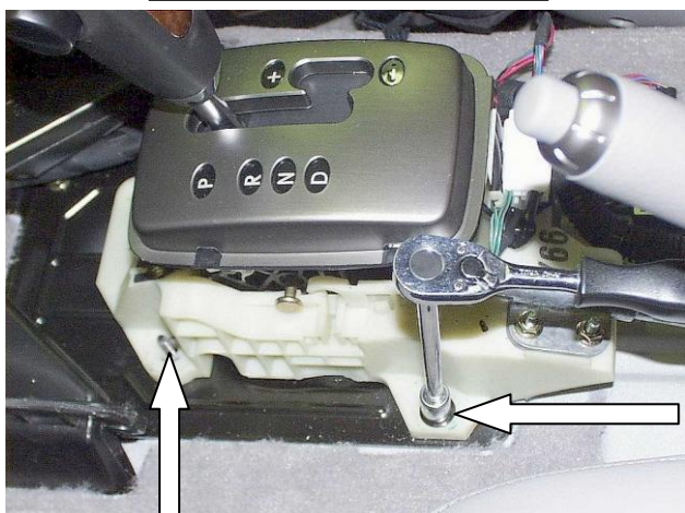
Открутить 2 гайки
