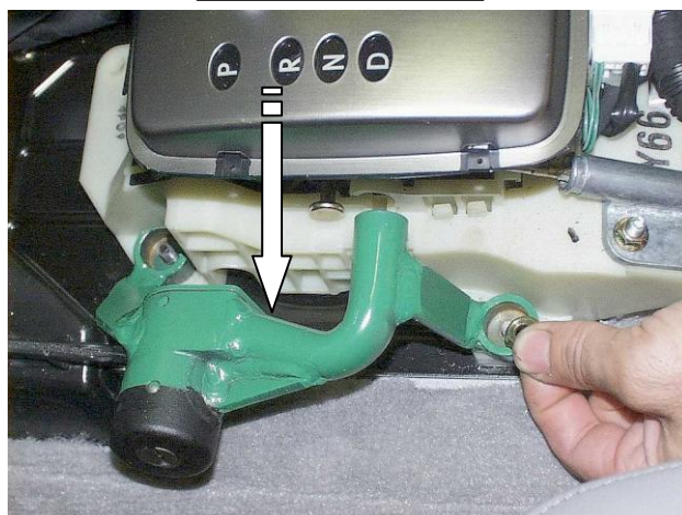
Установить замок на шпильки
