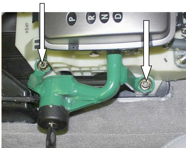
Закрутить 2 гайки
