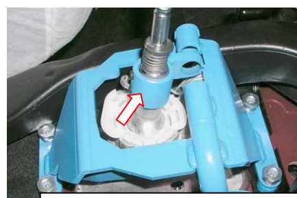
Установить хомут на рычаг переключения передач
