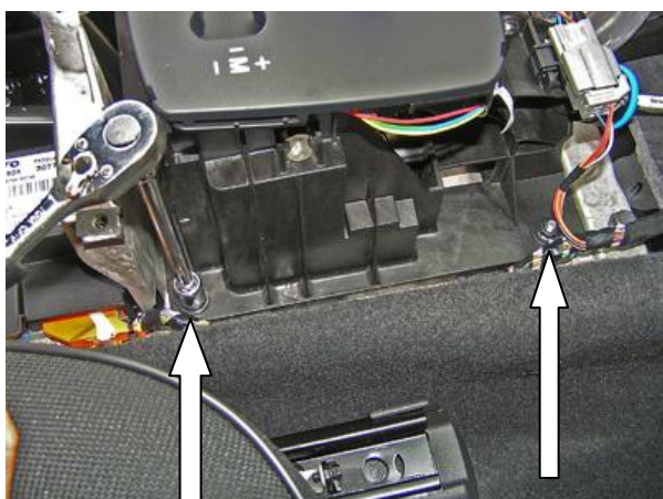
Открутить 2 гайки
