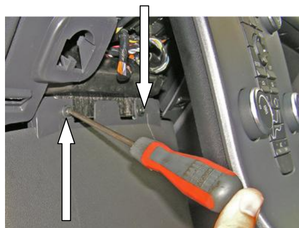
Открутить 2 самореза
