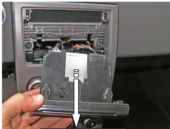
Снять магнитолу
