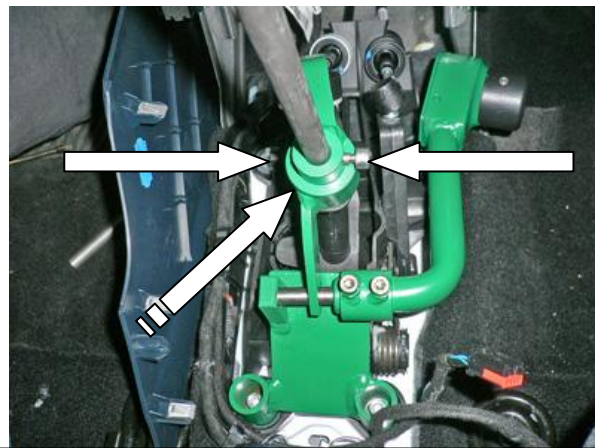
Установить хомут на рычаг переключения передач, зафиксировать 2 винтами
