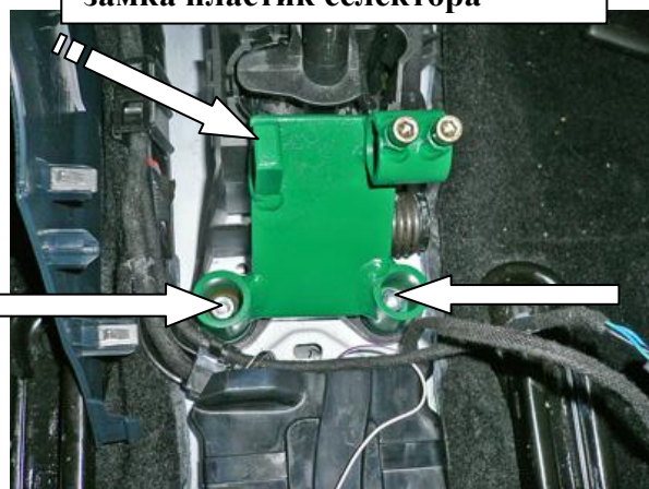
Установить кронштейн замка, закрутить 2 срывные гайки
