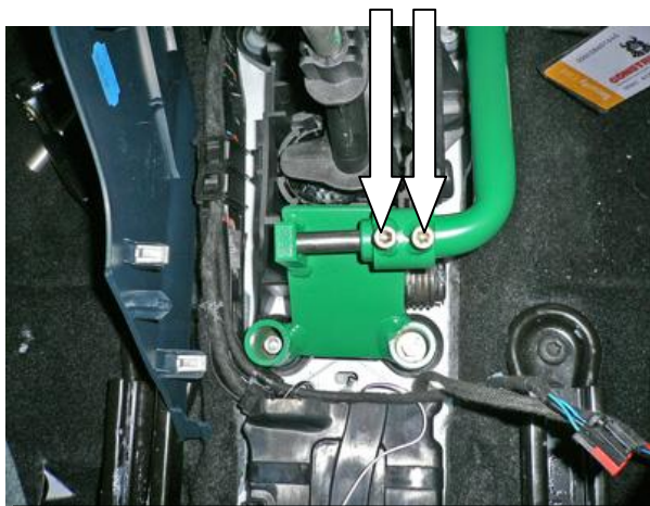
Зафиксировать трубу замка в кольце кронштейна замка 2 винтами
