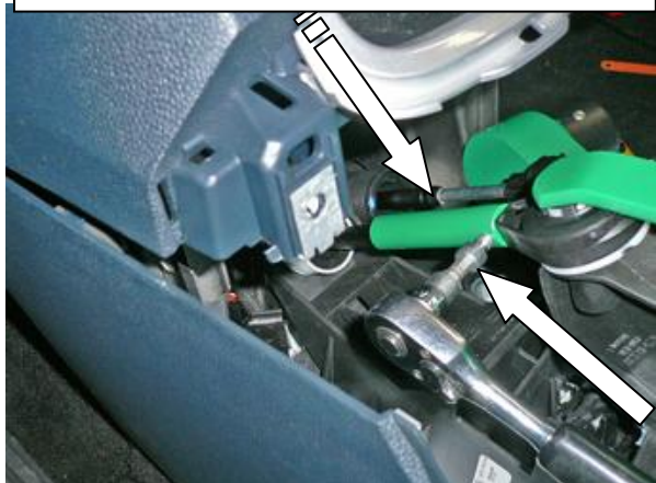
Установить защиту на тягу, зафиксировать винтом
