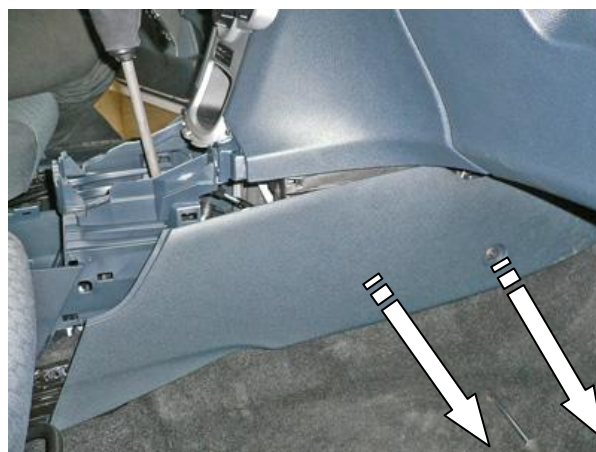
Вынуть клипсы, снять боковые крышки с обеих сторон
