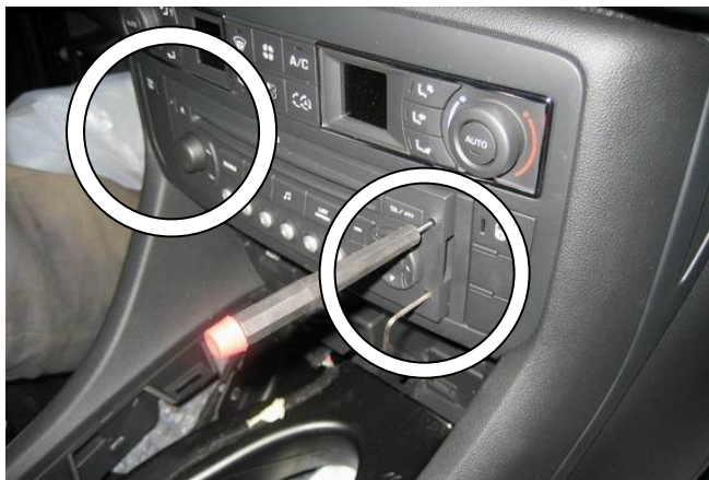
Нажать фиксаторы магнитолы в 4 гнездах
